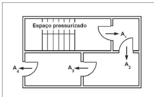
Figura 2: Trajetórias de escape do ar em série
