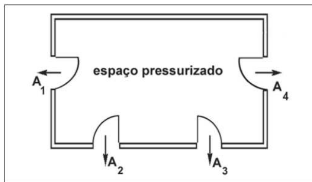
Figura 1: Trajetórias de escape do ar em paralelo
