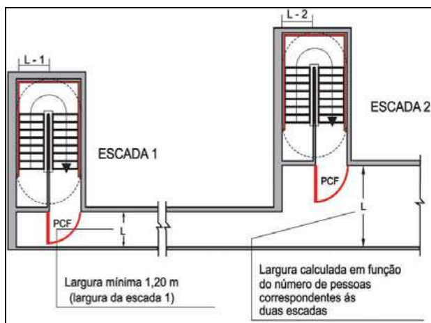
Figura 17: Dimensionamento de corredores de descarga
