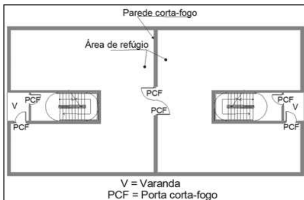
Figura 15: Desenho esquemático da área de refúgio
