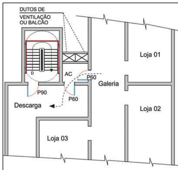
Figura 18: Acesso de galeria comercial à descarga
