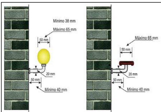
Figura 13: Pormenores de corrimãos
