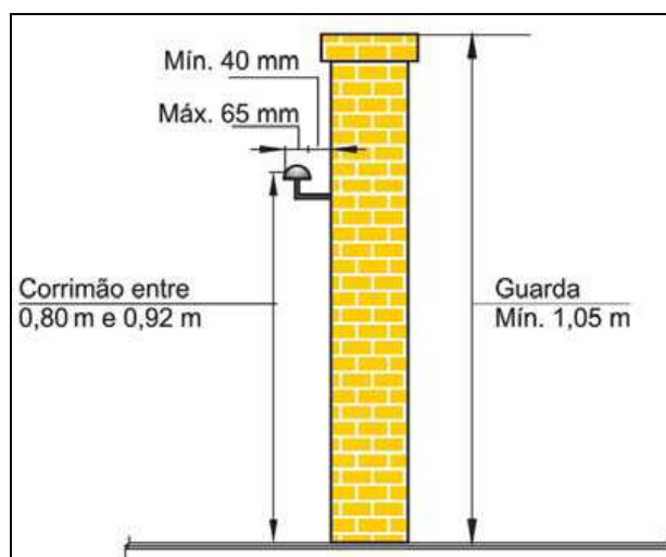
Figura 12: Dimensões de guardas e corrimãos
