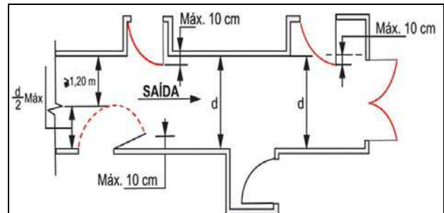
Figura 2: Abertura das portas no sentido de saída
