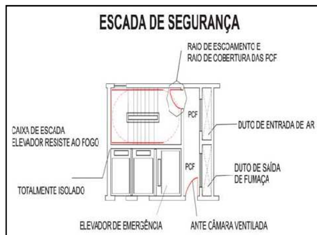
Figura 15: Escada e elevador à prova de fumaça
